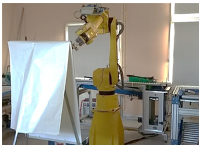
Photo de la cellule robotisée équipée d'un robot FANUC M-16iB. Possibilité d'y faire aussi bien des applications pédagogiques qu'industrielles.
